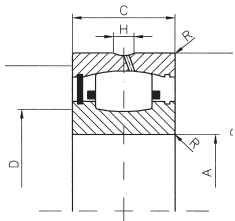
zylindrische Bohrung
