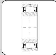
Pendelrollenlager McGill
